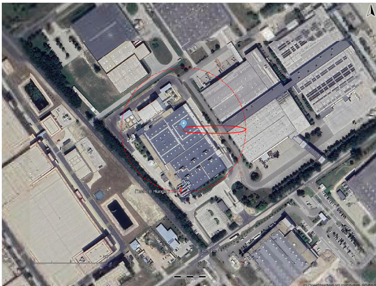
32. ábra - Alacsony hőmérsékletű raktár raktártüze (HF terjedése, D1 légkör állapot)
